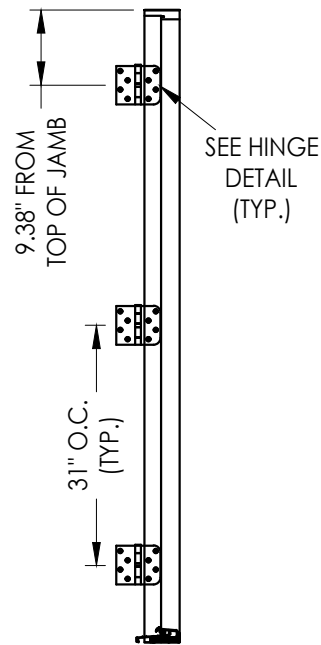
HINGE JAMB
